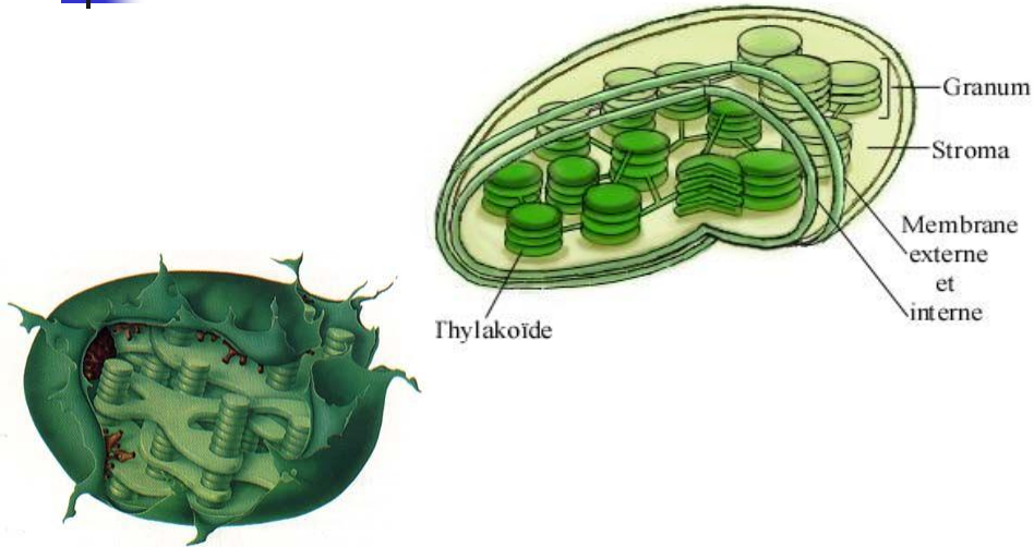
Chloroplaste
